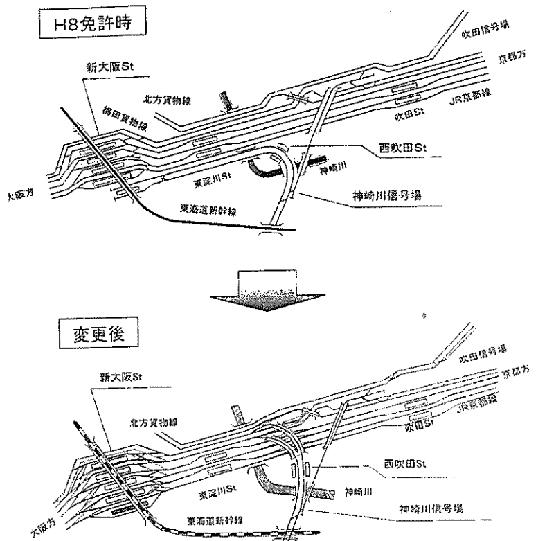
おおさか東線路線略図(変更区間)
